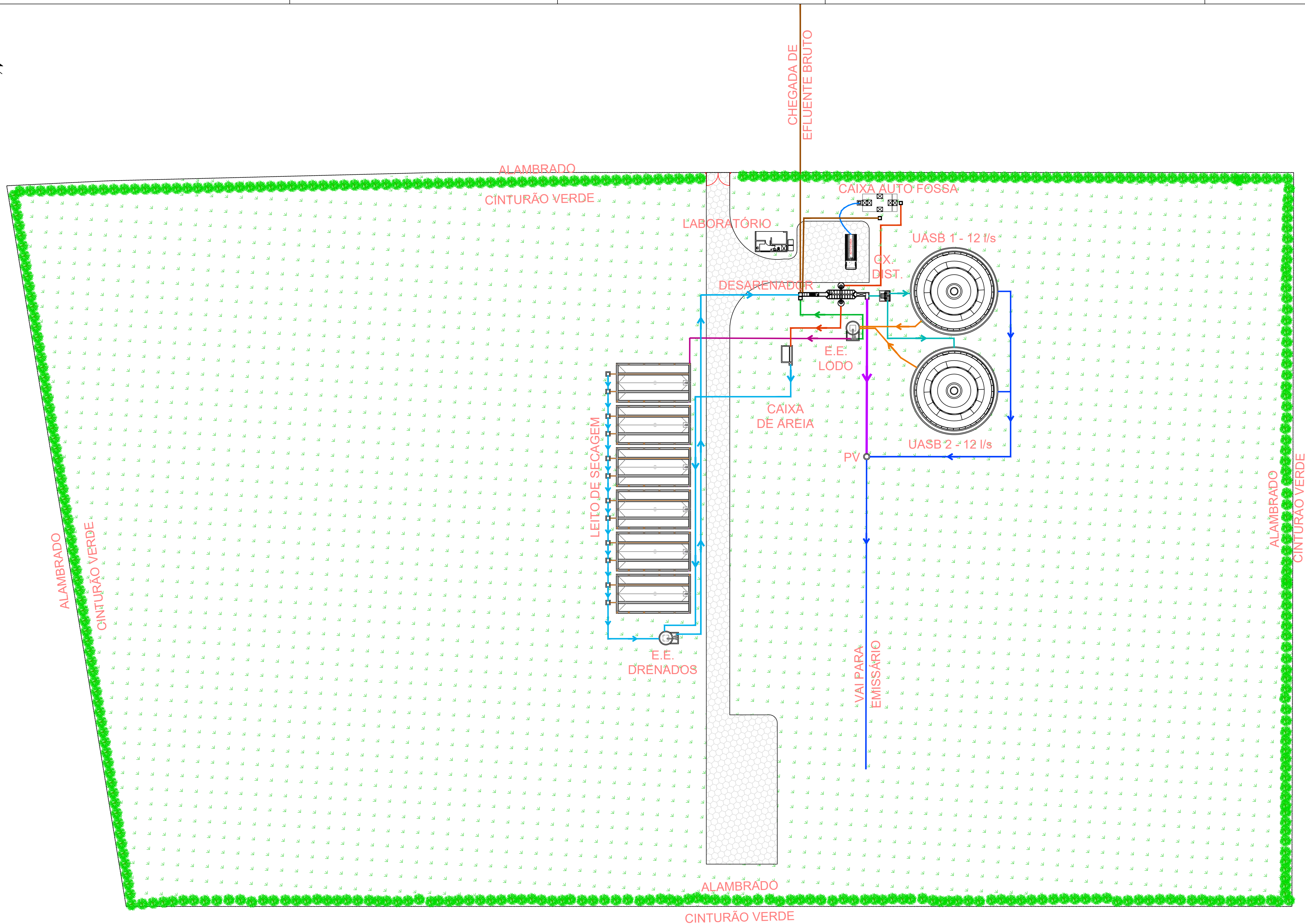
IMPLANTAÇÃO ESCALA 1:350
