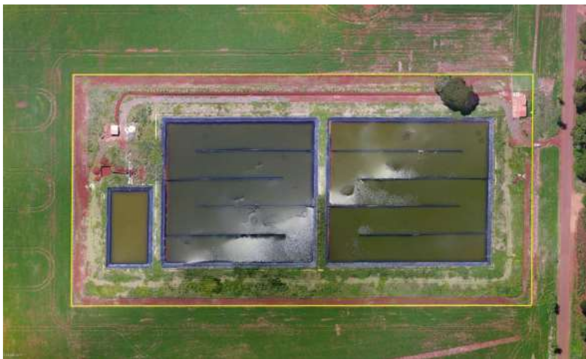
Figura 2: Vista aérea da ETE Douradina, Douradina, MS.
