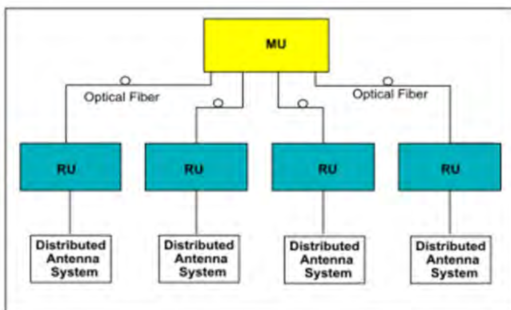
Figura 2.9 - Arquitetura para o sistema Wi-Fi.
