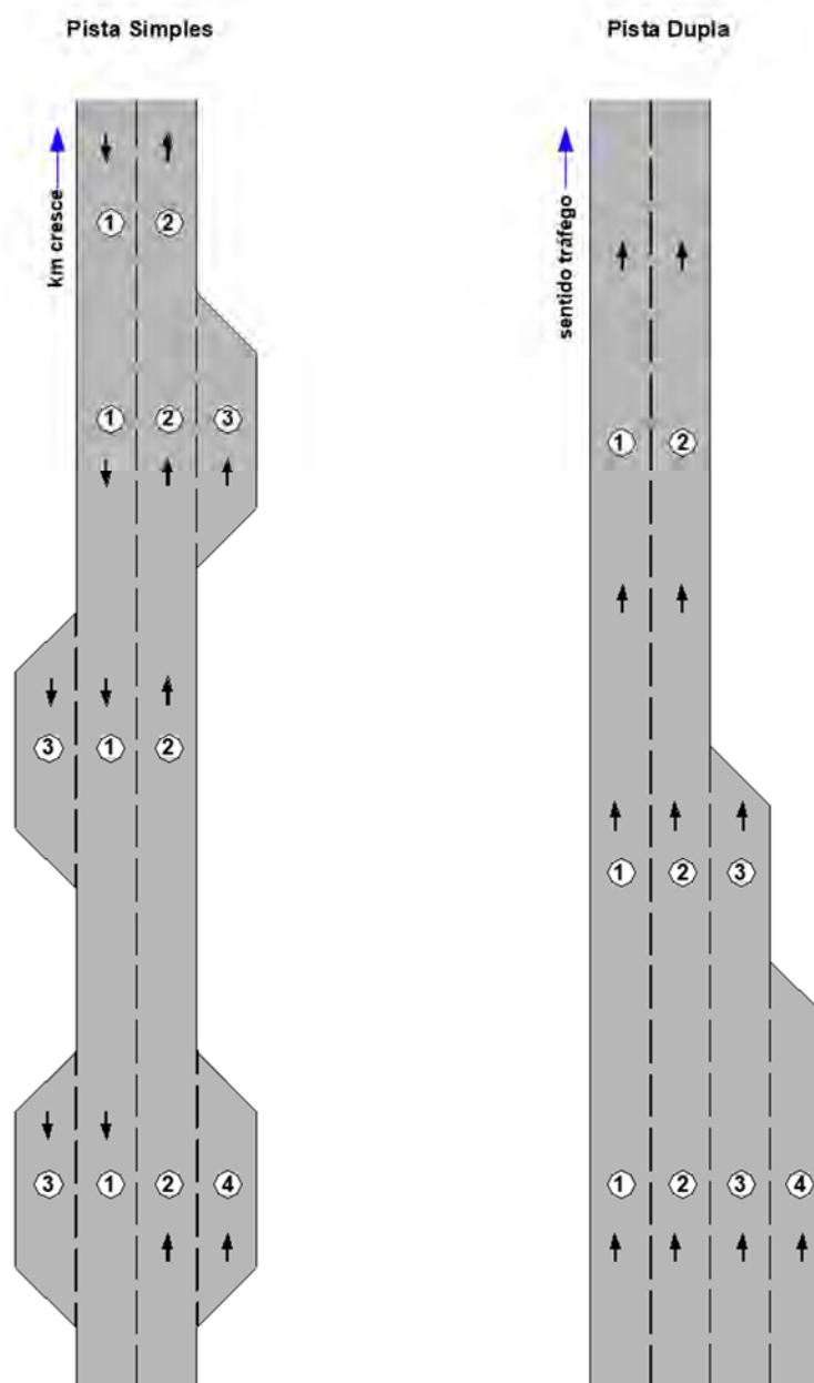
Figura 4.2 – Convenção da Numeração das Faixas de Tráfego.
