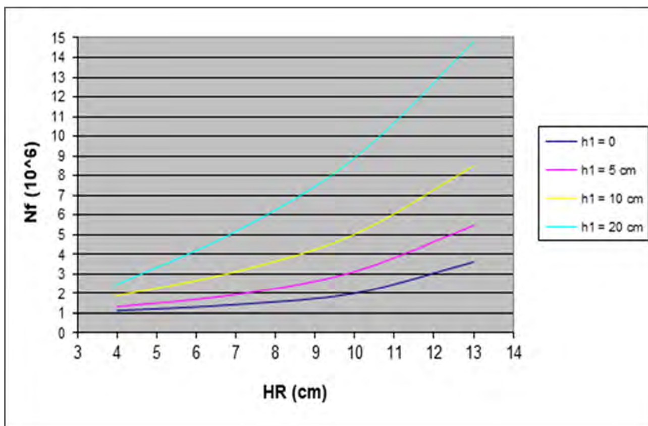
Figura 4.7 - Vida de fadiga de camada asfáltica de recapeamento.
